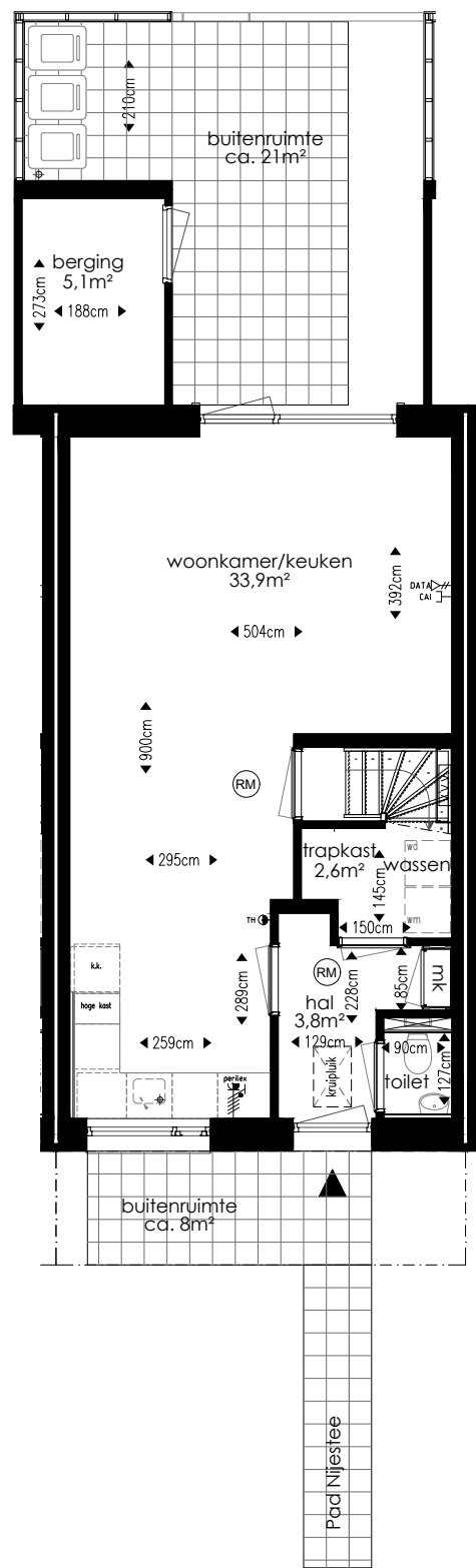
Begane grond
